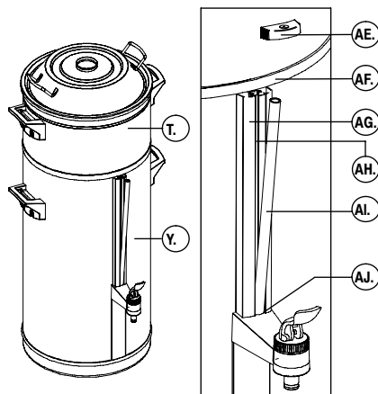
Fig. 10 Limpieza del indicador de nivel
